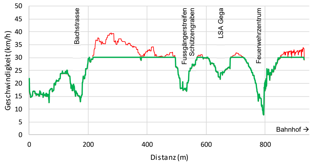
Abb. 3: Geschwindigkeitsprofil des Abschnitts (arithmetisch Mittel). Rote Linie: gemessene Geschwindigkeiten Grüne Linie: Theoretisches Geschwindigkeitsprofil mit Tempo 30
