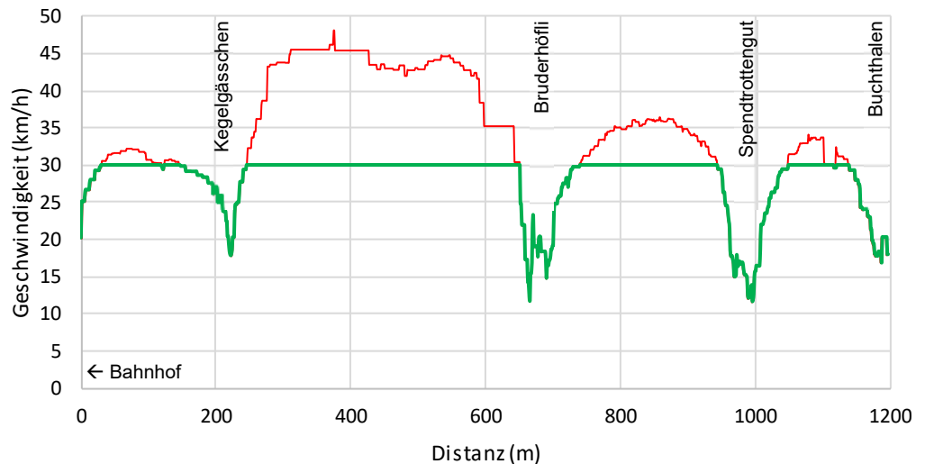
Abb. 4: Geschwindigkeitsprofil des Abschnitts (arithmetisch Mittel). Rote Linie: gemessene Geschwindigkeiten Grüne Linie: Theoretisches Geschwindigkeitsprofil mit Tempo 30
