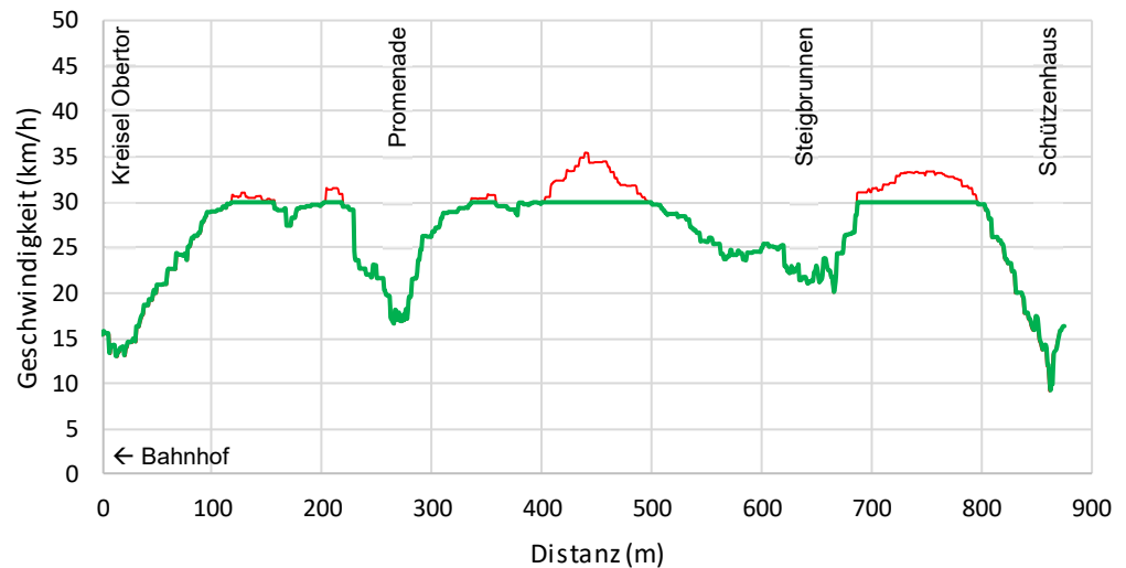
Abb. 10: Geschwindigkeitsprofil des Abschnitts (arithmetisch Mittel). Rote Linie: gemessene Geschwindigkeiten Grüne Linie: Theoretisches Geschwindigkeitsprofil mit Tempo 30
