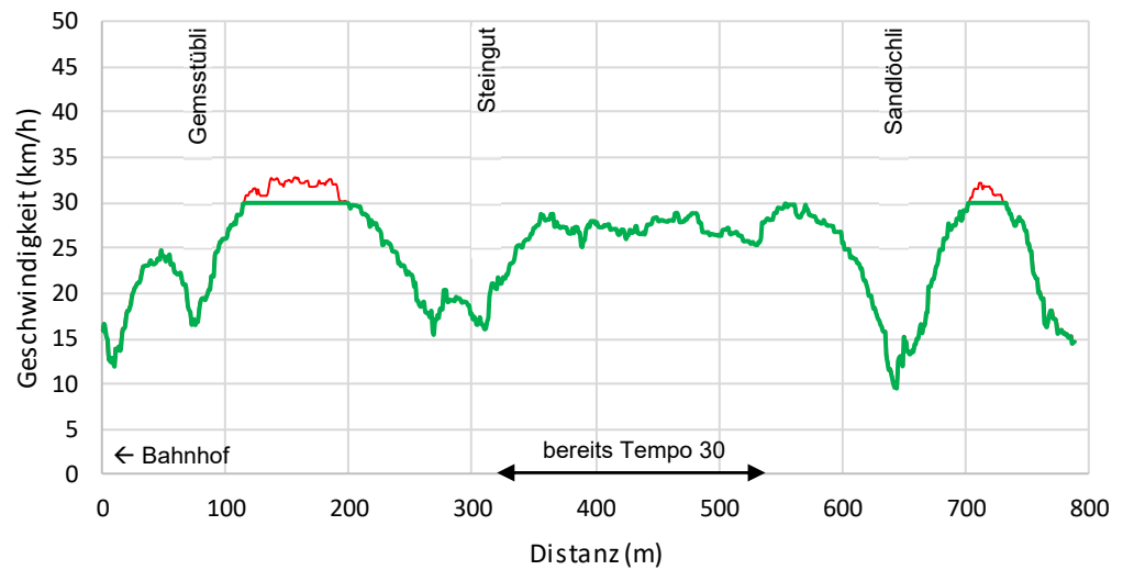
Abb. 7: Geschwindigkeitsprofil des Abschnitts (arithmetisch Mittel). Rote Linie: gemessene Geschwindigkeiten Grüne Linie: Theoretisches Geschwindigkeitsprofil mit Tempo 30
