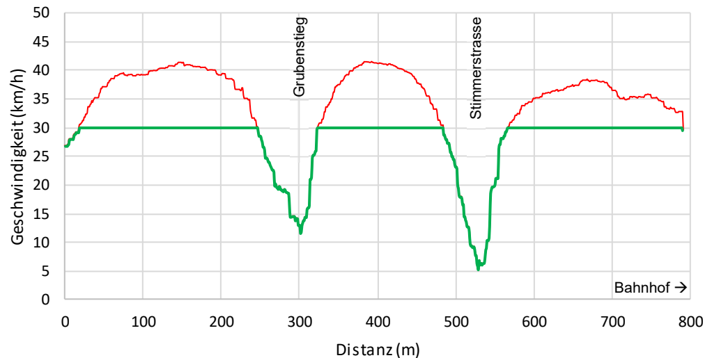
Abb. 6: Geschwindigkeitsprofil des Abschnitts (arithmetisch Mittel).
