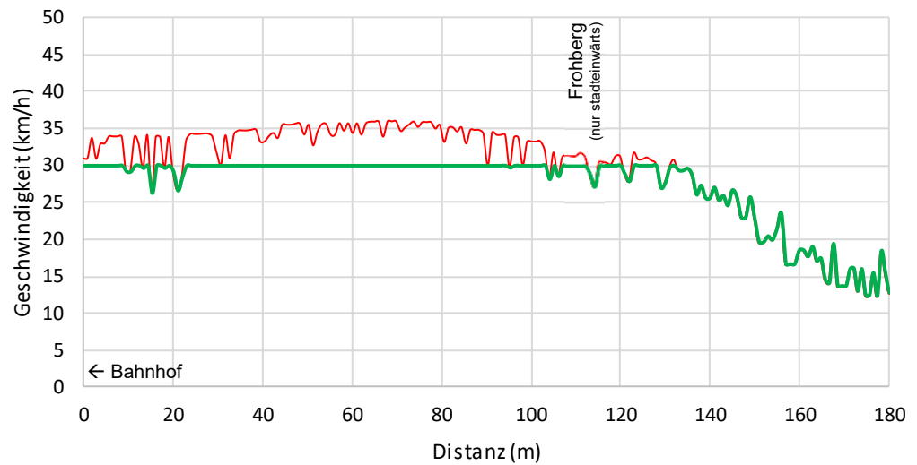
Abb. 5: Geschwindigkeitsprofil des Abschnitts (arithmetisch Mittel).
