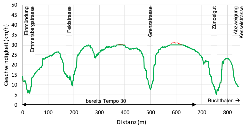
Abb. 2: Geschwindigkeitsprofil des Abschnitts (arithmetisch Mittel). Rote Linie: gemessene Geschwindigkeiten Grüne Linie: Theoretisches Geschwindigkeitsprofil mit Tempo 30
