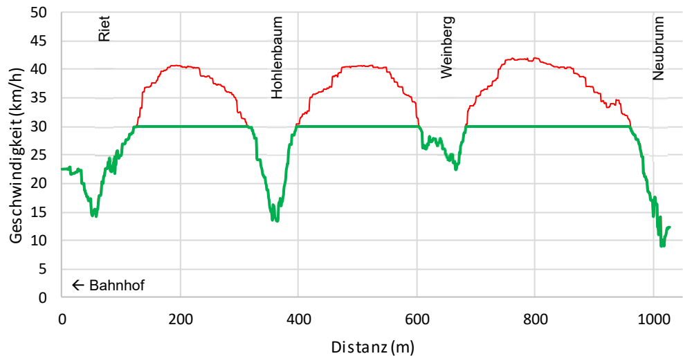
Abb. 8: Geschwindigkeitsprofil des Abschnitts (arithmetisch Mittel). Rote Linie: gemessene Geschwindigkeiten Grüne Linie: Theoretisches Geschwindigkeitsprofil mit Tempo 30
