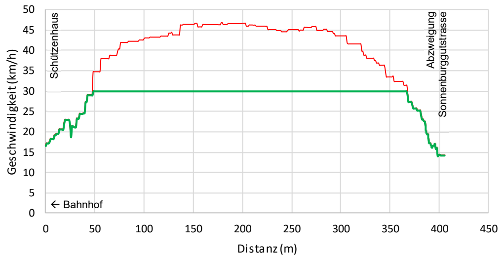
Abb. 9: Geschwindigkeitsprofil des Abschnitts (arithmetisch Mittel). Rote Linie: gemessene Geschwindigkeiten Grüne Linie: Theoretisches Geschwindigkeitsprofil mit Tempo 30
